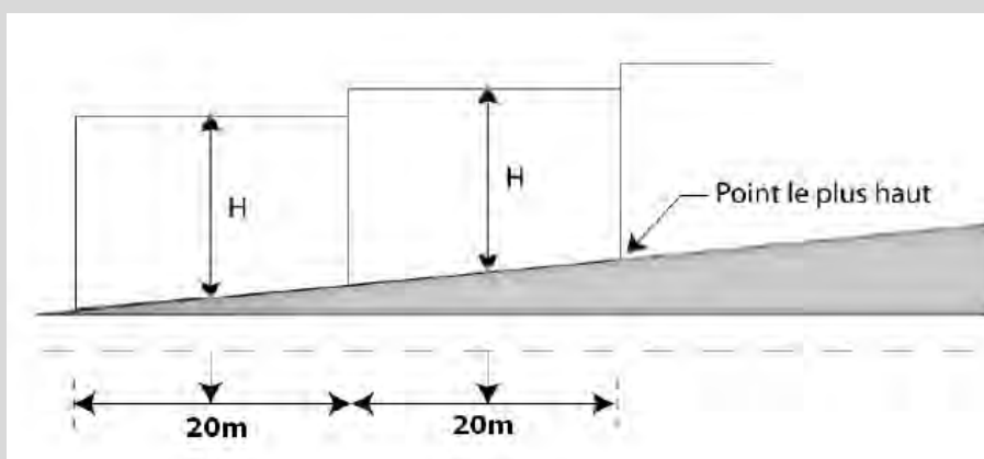
Calcul des hauteurs par rapport au terrain naturel
